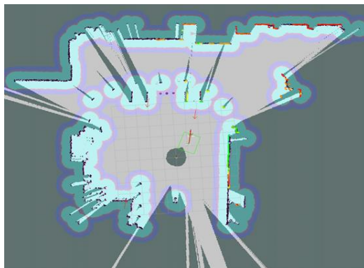
図 1 レーザーセンサーによる周辺環境の認識
