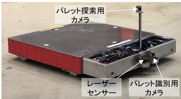
写真 1 低床式 AGV とセンサー・カメラ
